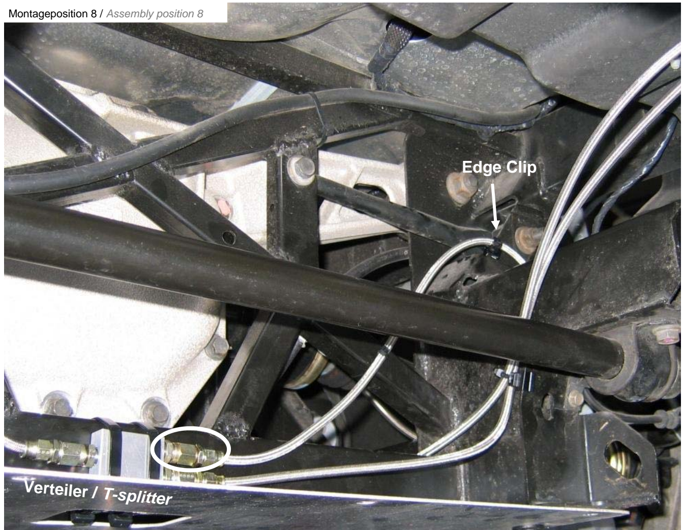
Edge Clip
