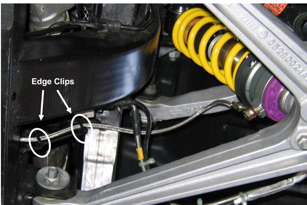
Edge Clip
