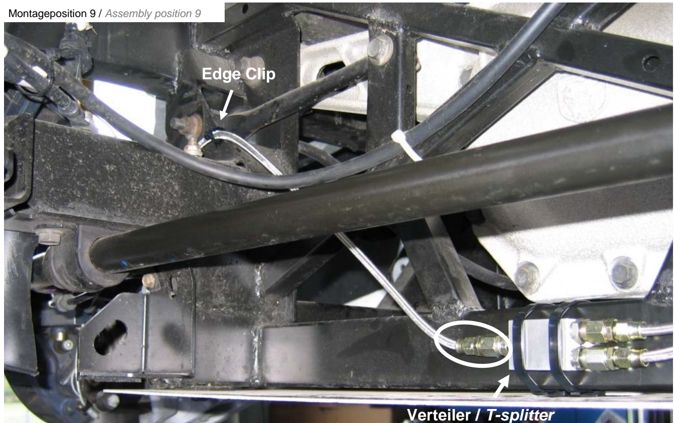
Edge Clip
